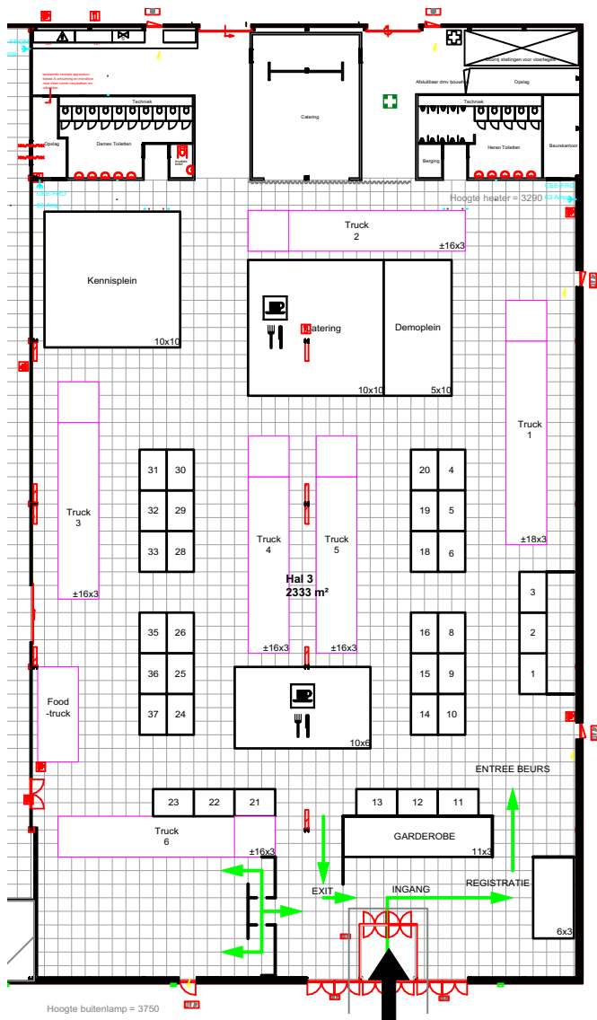
Plattegrond (1:500 A3)
